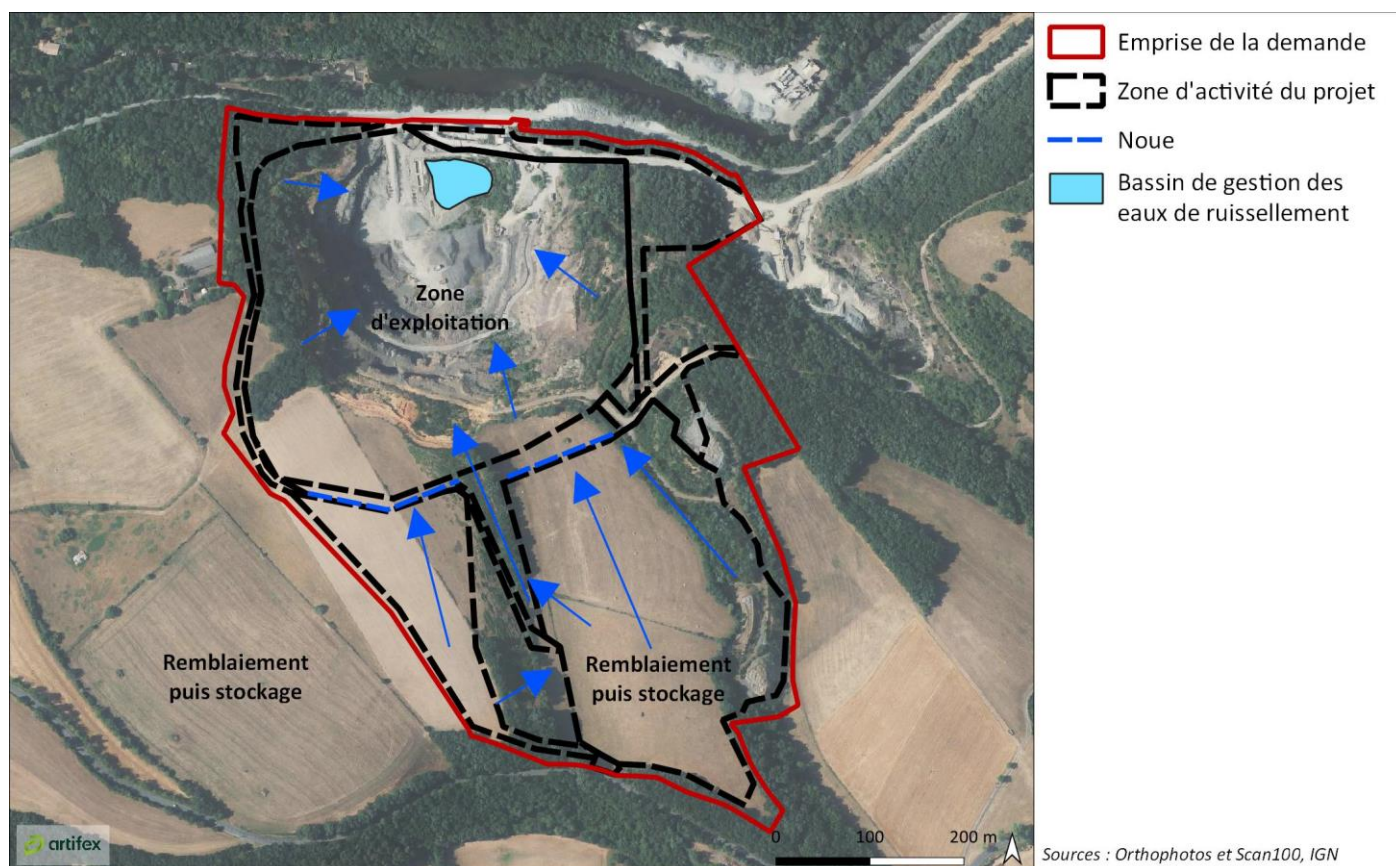
Illustration 27 : Gestion des eaux de ruissellement sur le site du Rivet Réalisation : ARTIFEX 2023
