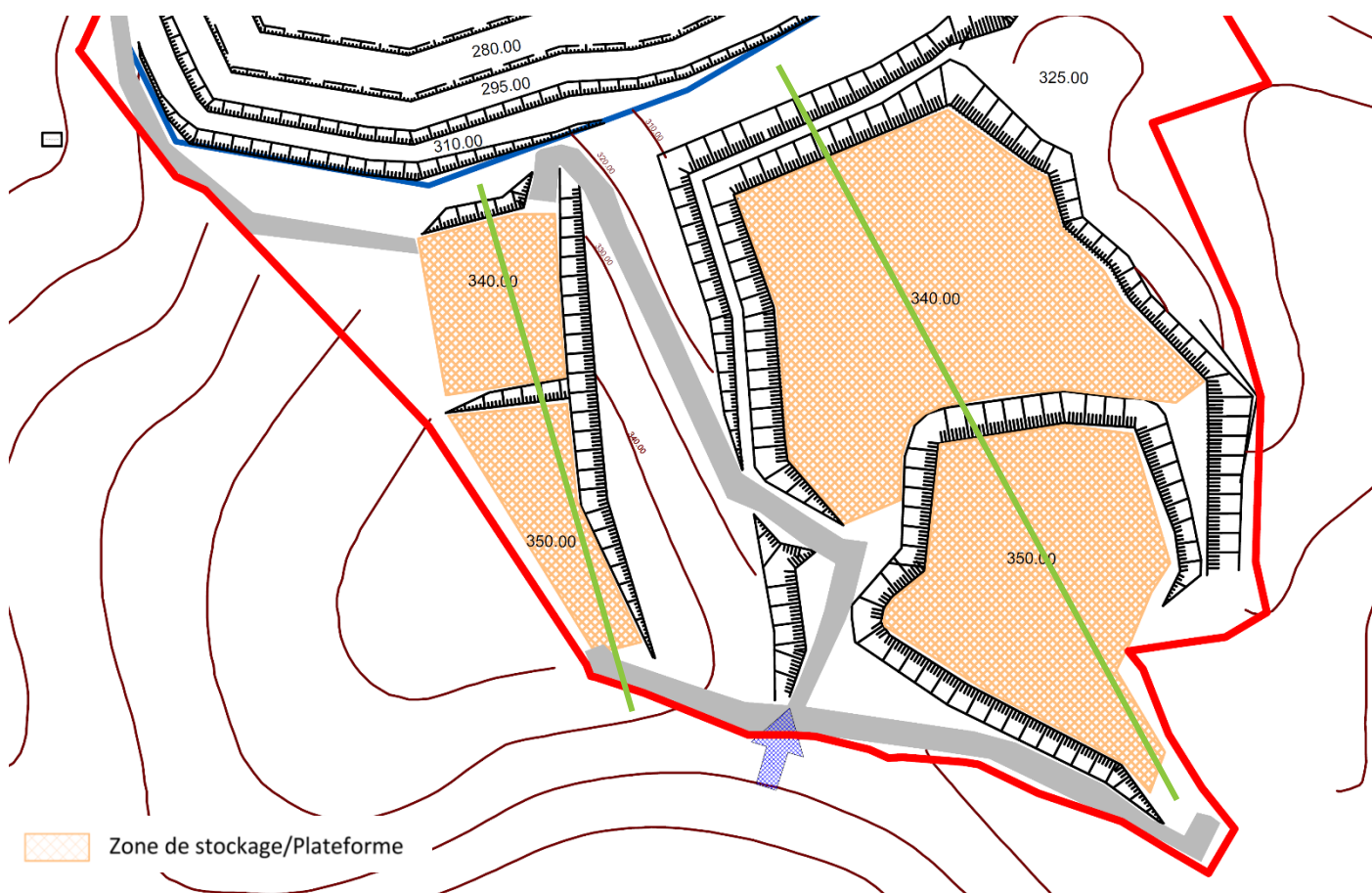
Illustration 18 : Localisation des plateformes de stériles projetées / coupe de principe sans échelle
