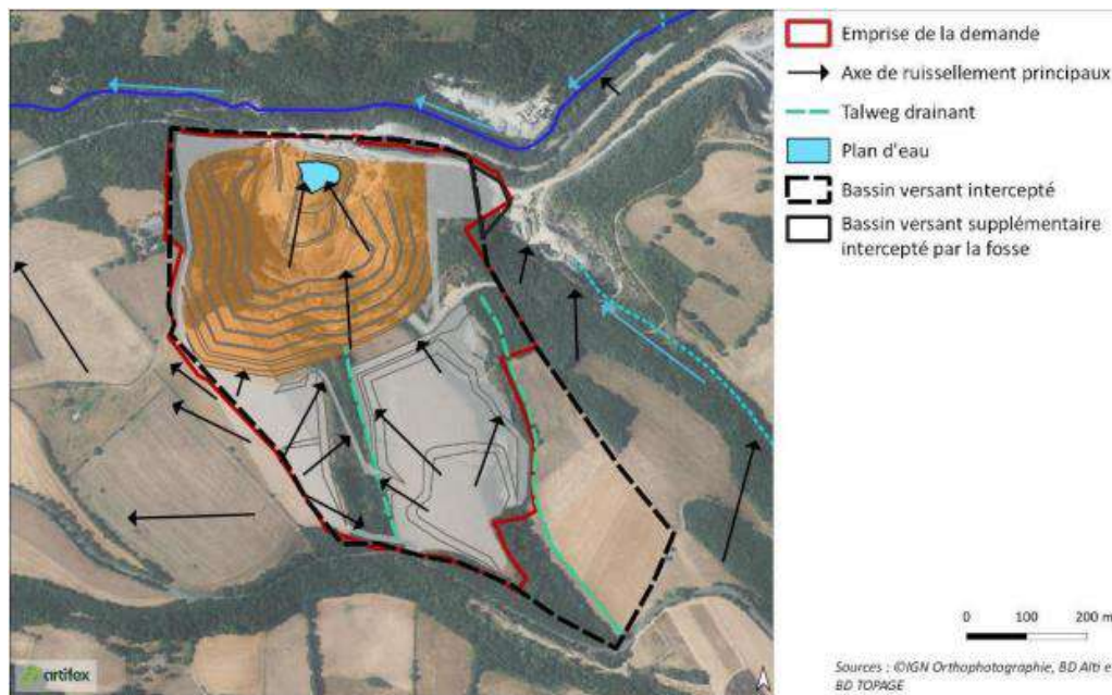
Bassin versant du site du projet (BE Artifex – en charge de l'élaboration de l'évaluation environnementale projet)
