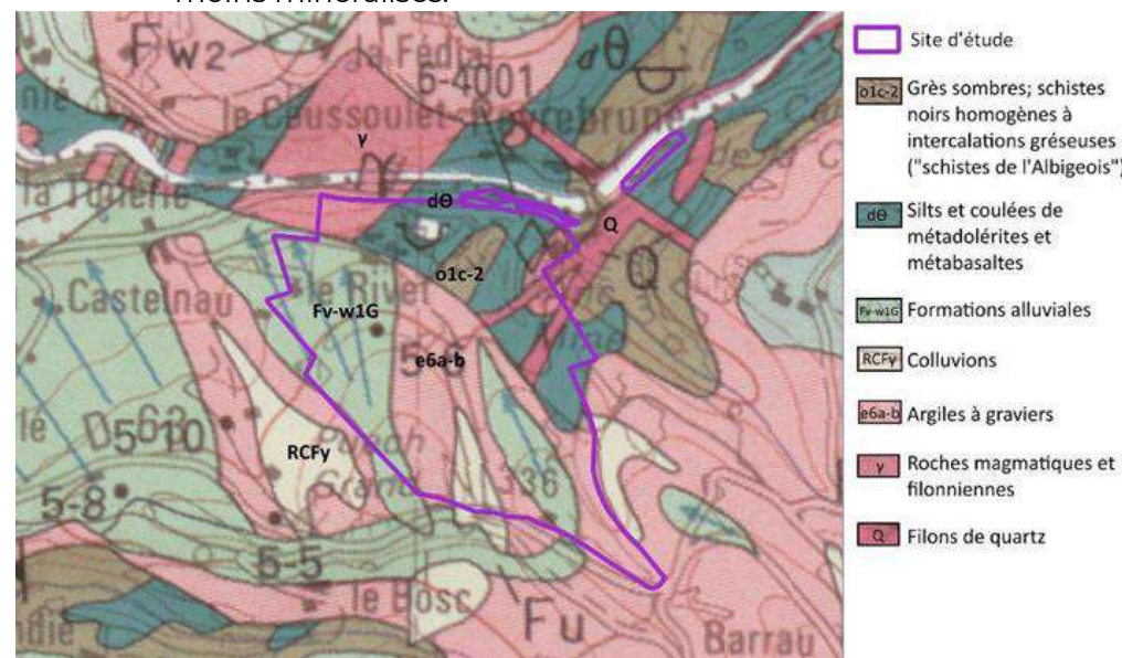
Carte géologique (BE ARTIFEX- en charge de l'élaboration de l'évaluation environnementale projet)
